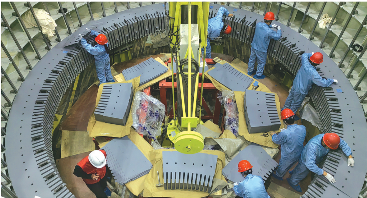
国网新疆阜康抽水蓄能电站施工人员正在进行1号机组定子铁芯叠片工作。
