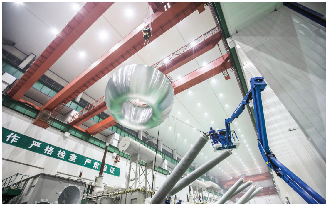
特变电工新疆输变电科技产业园新疆变压器厂特高压试验大厅,工人们正在为特高压产品安装套管。 李宏吉 摄
