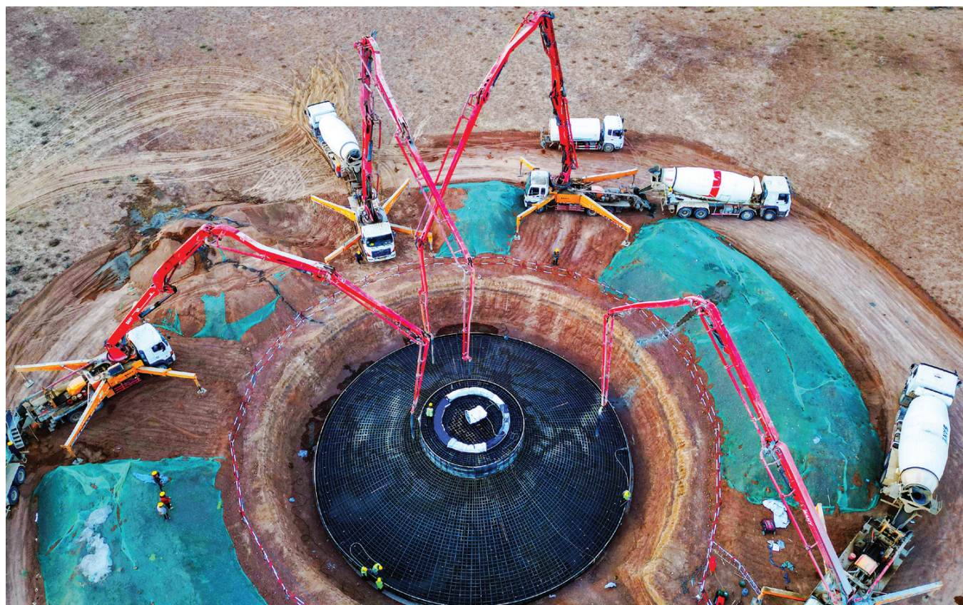
9月26日,在木垒县四十个井子风电规划区第六风电场的昌吉绿能新能源有限公司400兆瓦风电及配套220千伏汇集站项目EPC总承包项目施工现场,中煤建筑安装工程集团有限公司新疆分公司的工人们正在浇筑风机基础。
